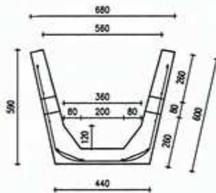
PRZEKRÓJ POPRZECZNY
