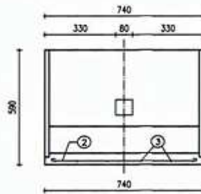
PRZEKRÓJ PODŁUŻNY
